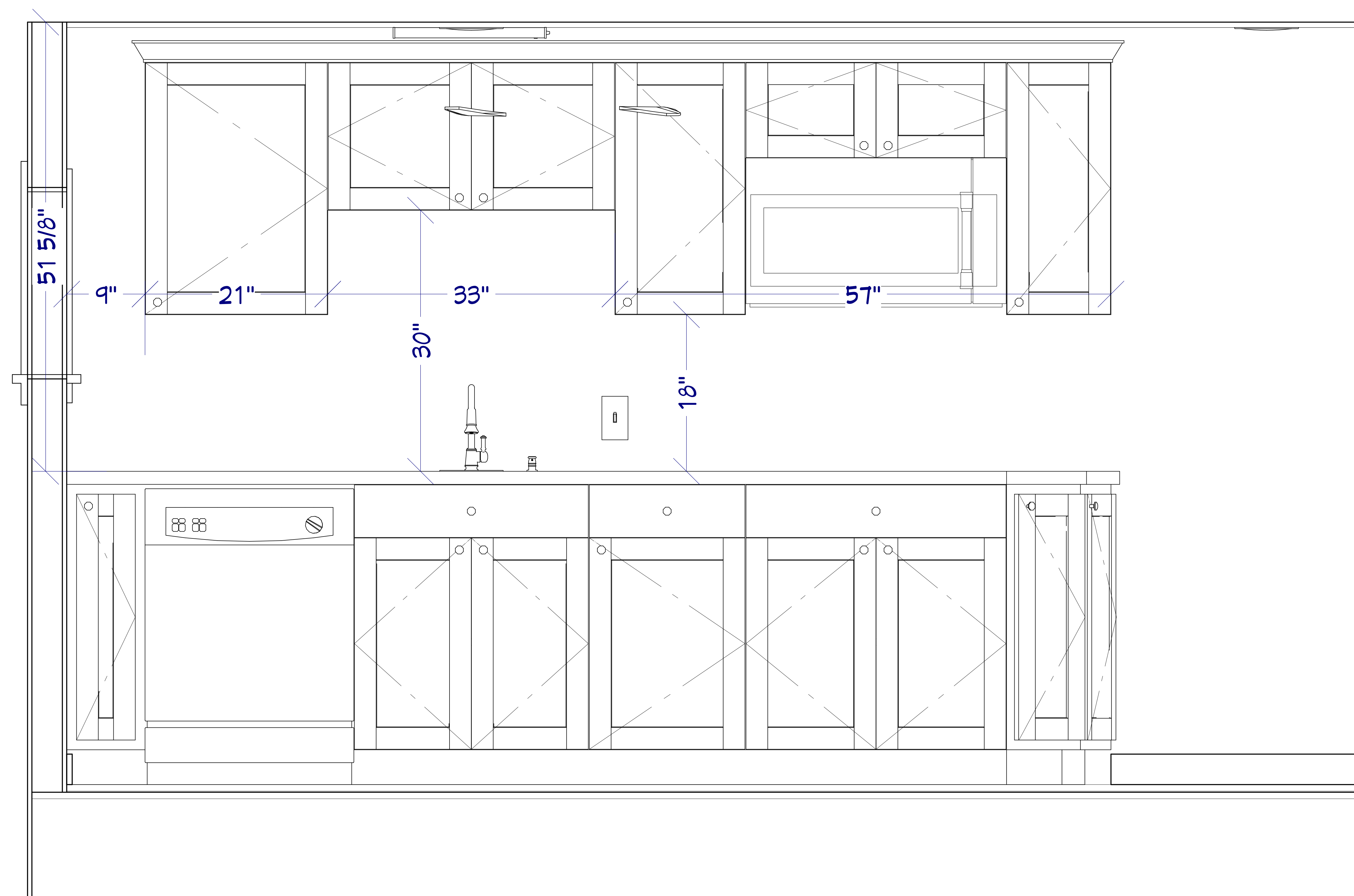
Elevation 3
