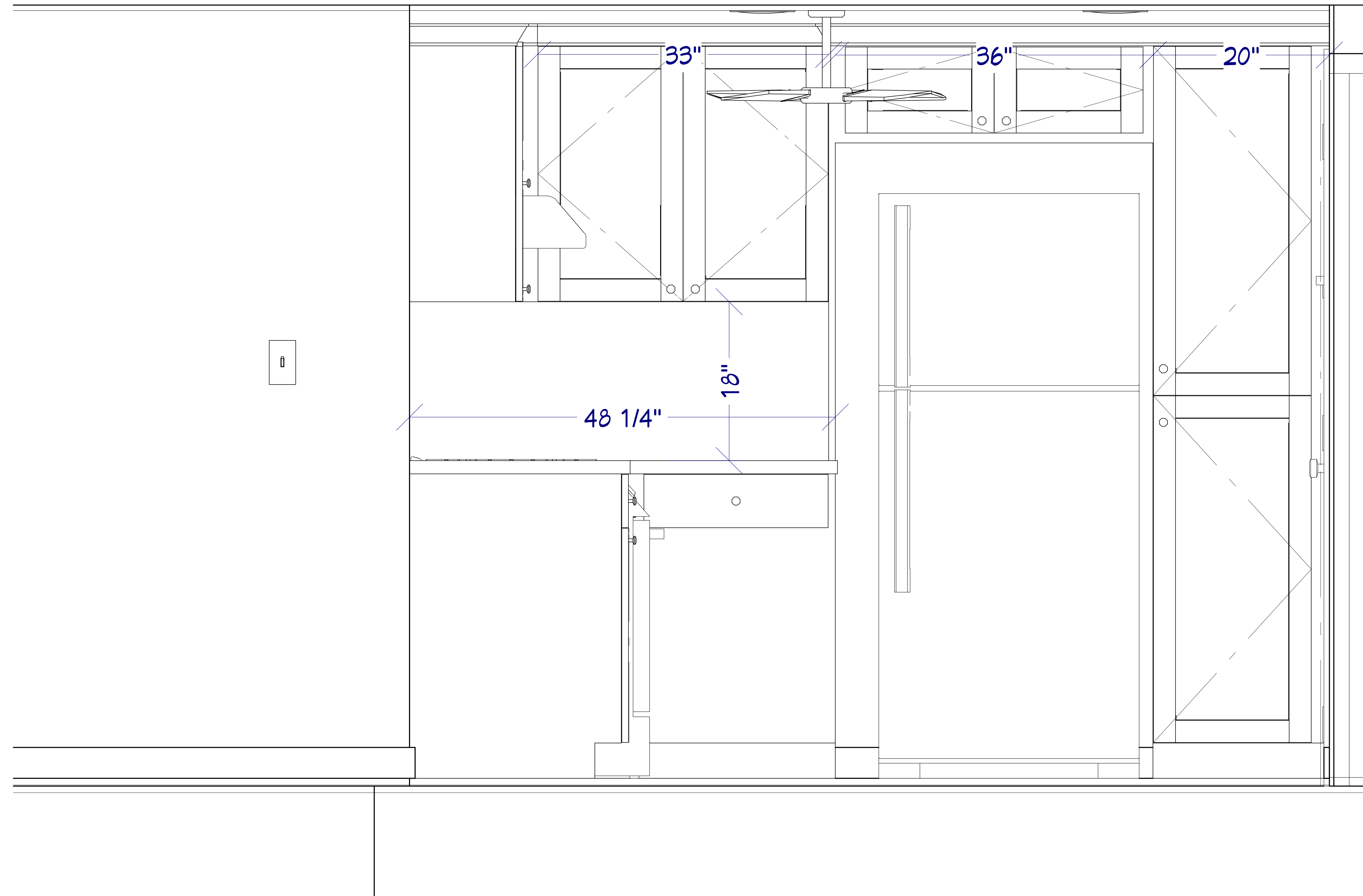
Elevation 1
