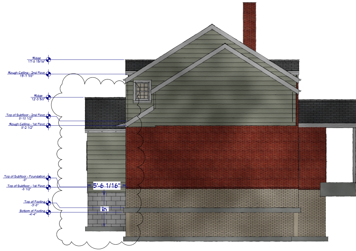
Elevation 4
