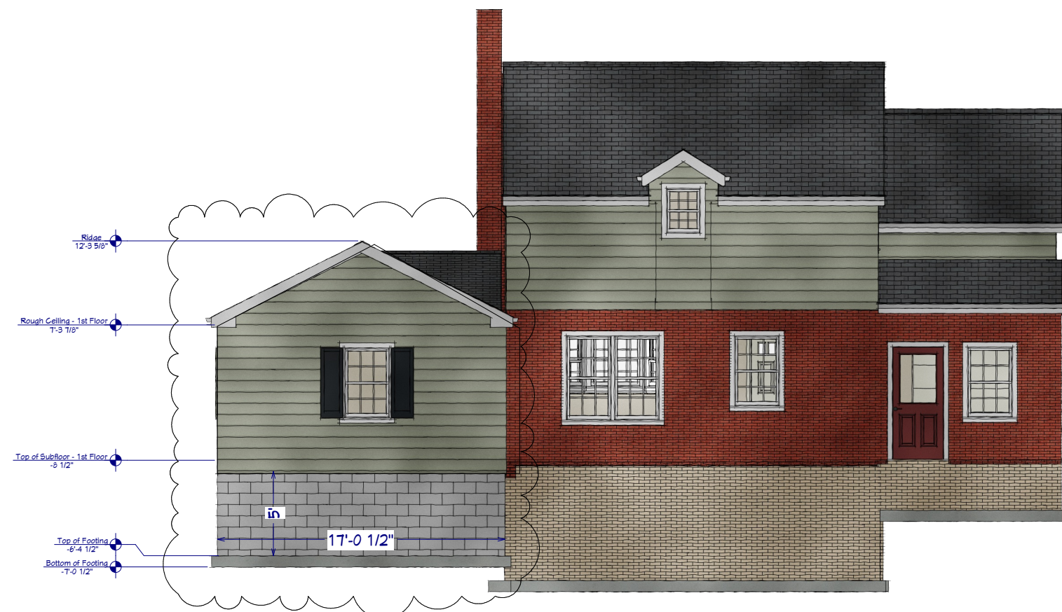
Elevation 1
