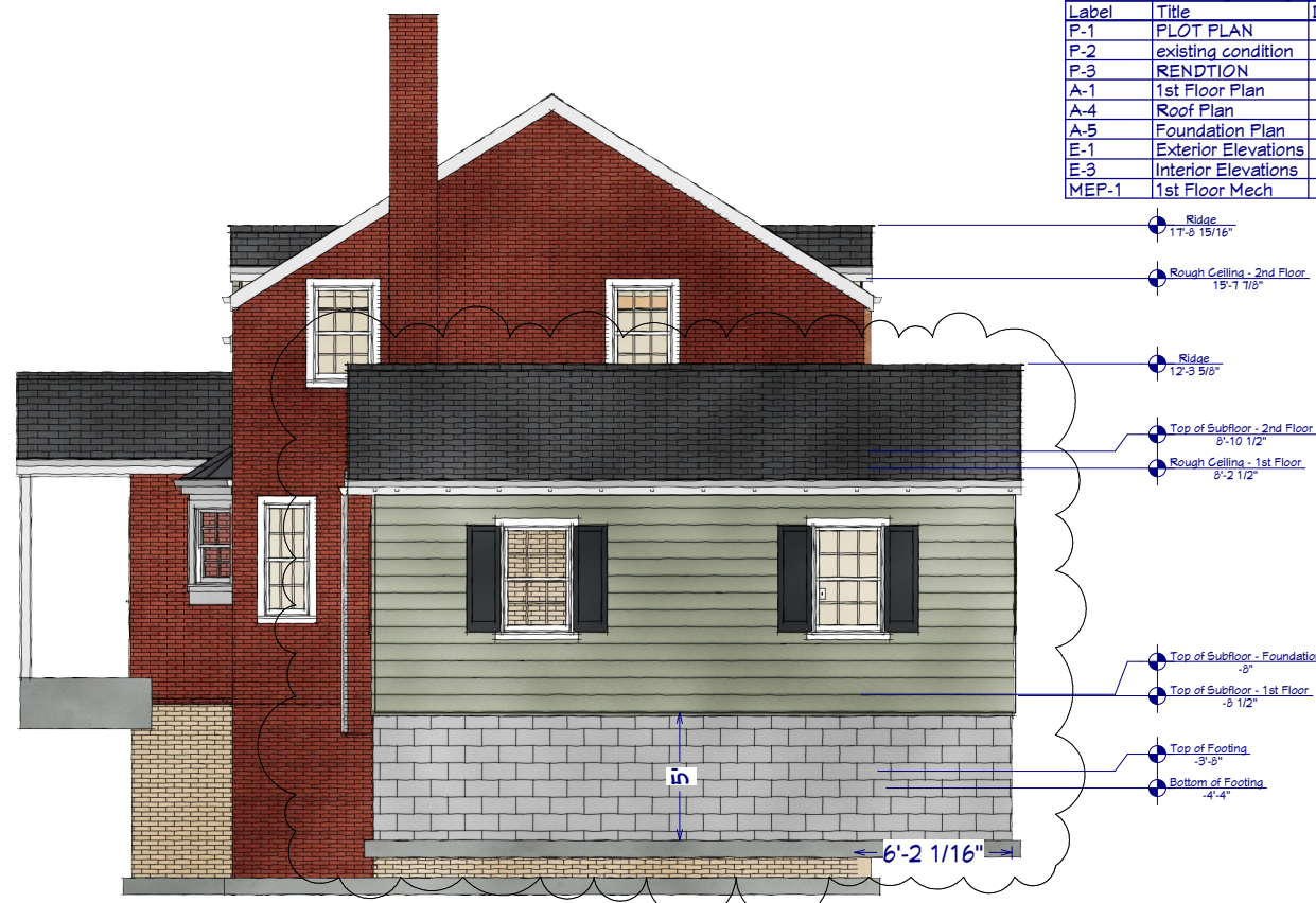
Elevation 2
